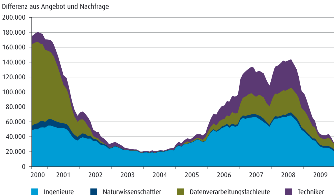
Abb. 3.7 MINT-Fachkräftemangel 2000–2009
